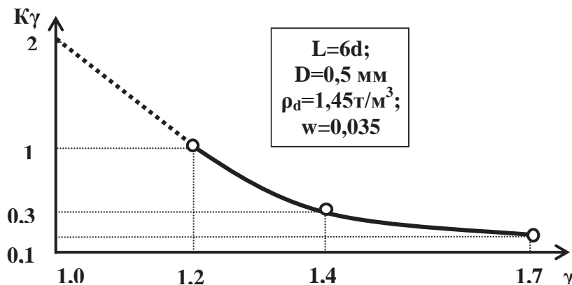
Рис. 2 – Залежність коефіцієнта K_{\gamma_k} від рівня навантаження на «існуючу» палу
