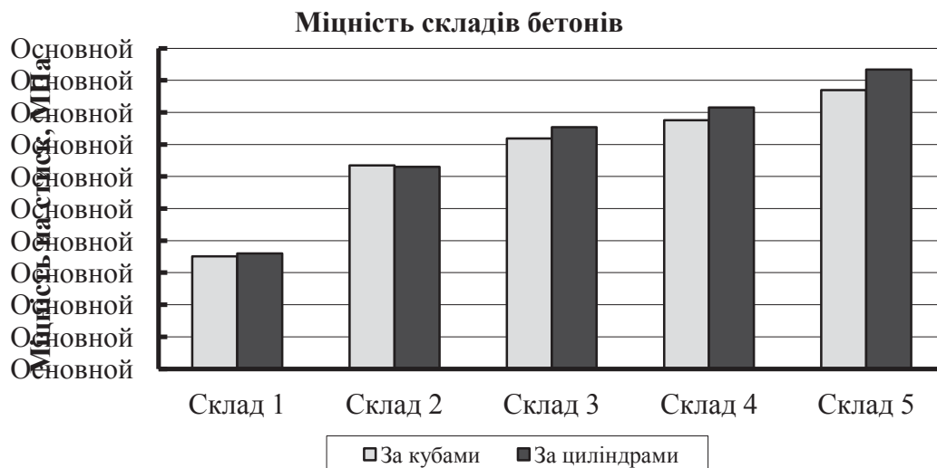
Рис. 1 – Міцність складів бетонів визначена на зразках-кубах та циліндрах
