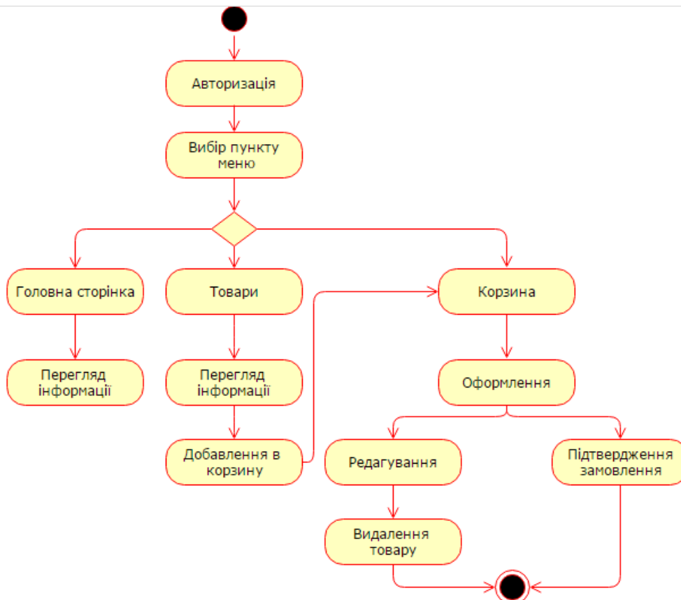
Рис. 5. Діаграма активності
