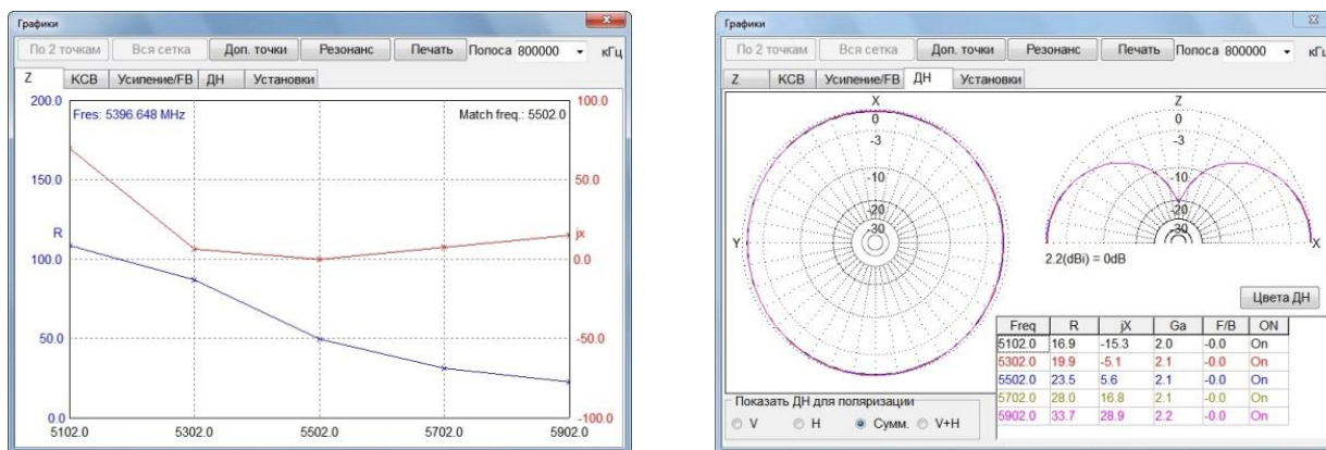
Рис. 9. Параметри масштабованої антени № 5
