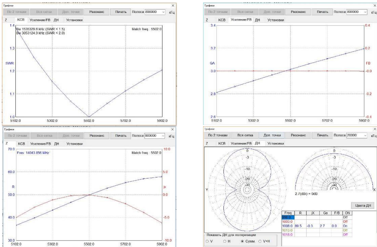
Рис. 7. Параметри масштабованої антени № 3
