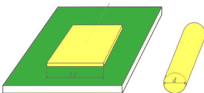
Рис. 1. Співвідношення мікросмужкового елемента та провідного вібратору
