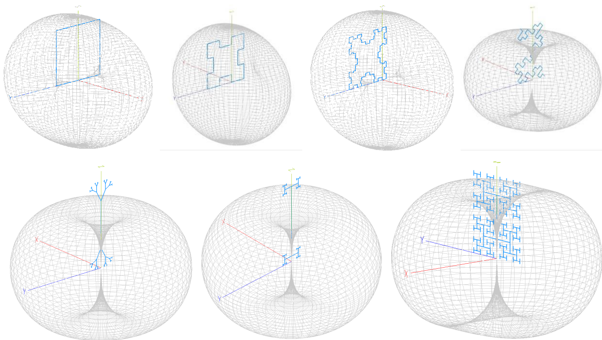
Рис. 4. Результуючі 3D ДС антен, що отримані в MMANA-GAL
