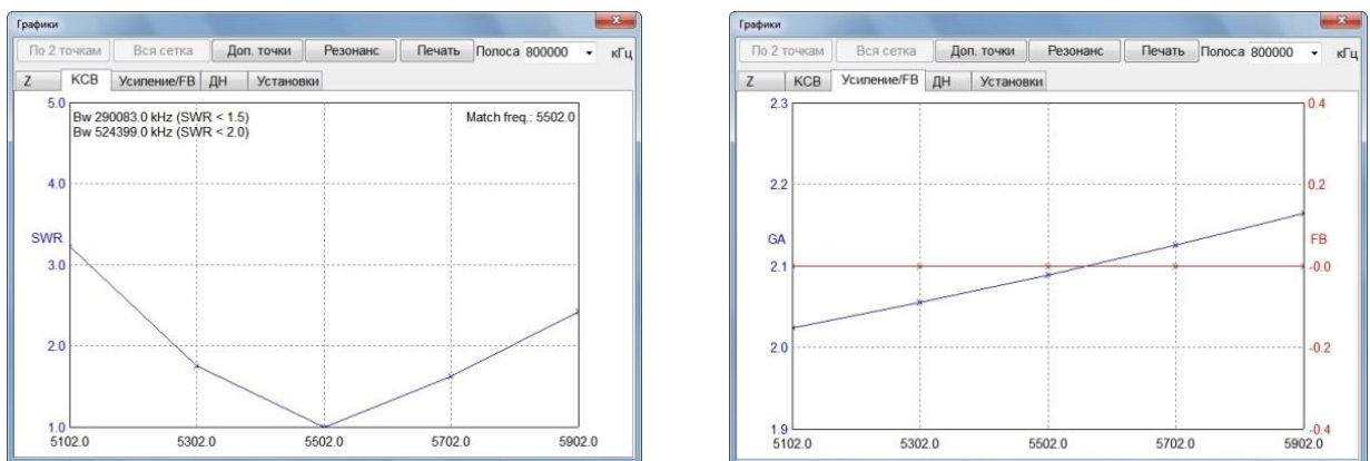
Рис. 8. Параметри базової антени № 5
